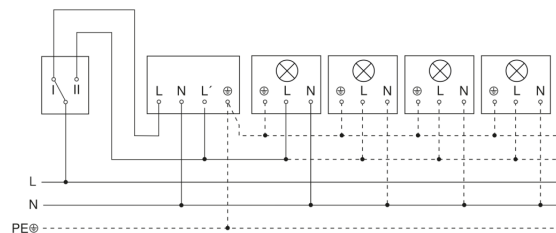
Aansluiting van 4-voudige drukknopkoppeling op DALI2 APC
